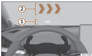
Afb. 4 In het gezichtsveld van de bestuurder: Proximity HUD ① en AR HUD ②.
