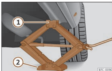
Afb. 217 Langsligger: plaatsing van de wagenkrik.
