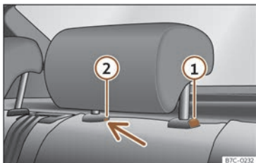
Afb. 91 Hoofdsteen achterin: verwijderen.
