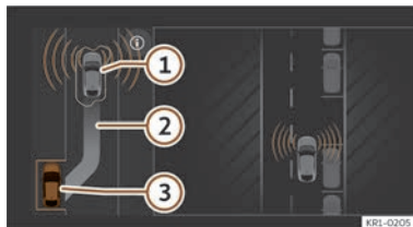
Afb. 147 Op het display van het infotainmentsysteem: positie om recht te parkeren.
