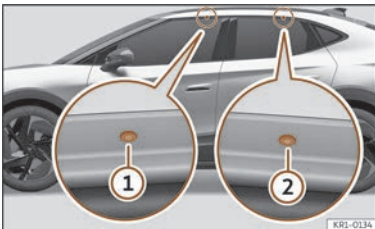
Afb. 181 Bevestigingspunten van de dwarsdragers voor het dakdragersysteem.
