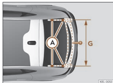
Afb. 187 Trekhaak: maten en bevestigingspunten.
