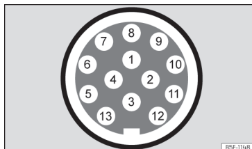
Afb. 182 Schematische weergave: toewijzing van de pinnen van het stopcontact voor de aanhangwagen.
