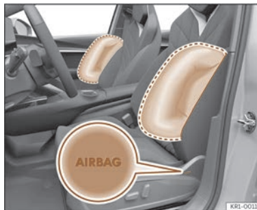
Afb. 33 Zij-airbag in de bestuurders- en bijrijdersstoel.
