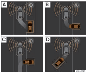
Afb. 145 Op het scherm van het infotainmentsysteem: aanduiding van de parkeermodi.
