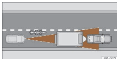
Afb. 129 Motorrijder die voor u rijdt, buiten de actieradius van de radarsensor.
