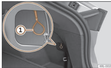
Afb. 64 Achter de afdekking: noodontgrendeling van de laadsteker.
