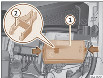
Afb. 202 In de voorruimte: deksel van de zekeringenhouder.
