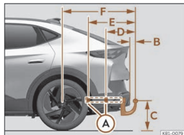
Afb. 186 Trekhaak: maten en bevestigingspunten.
