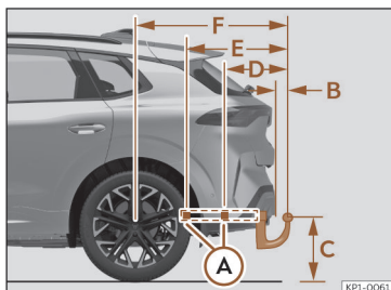
Afb. 200 Trekhaak: maten en bevestigingspunten.
