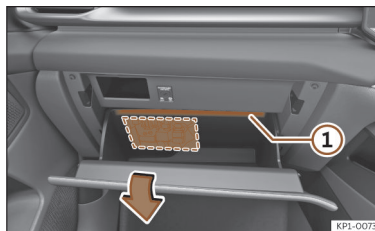
Afb. 218 Wagens met stuur rechts: zekeringenkast achter het dashboardkastje, aan bijrijderszijde.
