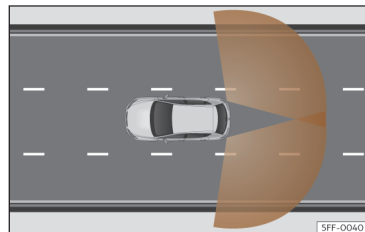
Afb. 128 Detectiegebieden van de sensoren.
