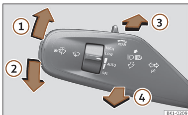
Afb. 103 Knipperlicht- en grootlichthendel.
