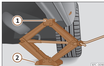
Afb. 245 Langsligger: plaatsing van de wagenkrik.
