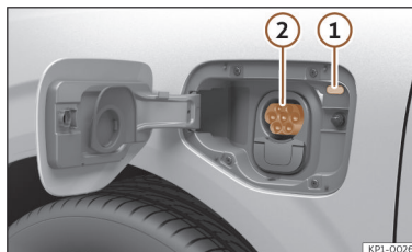
Afb. 58 Achter de laadklep van de accu linksvoor: Laadcontactdoos.
