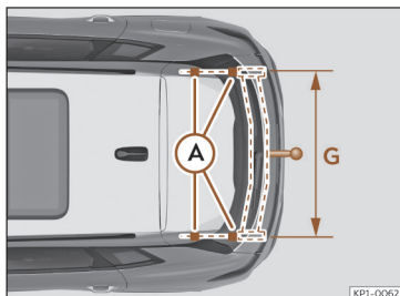
Afb. 201 Trekhaak: maten en bevestigingspunten.
