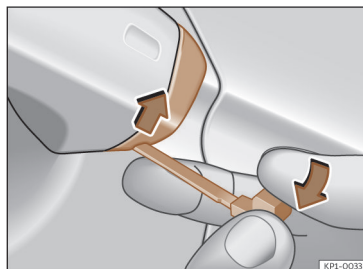
Afb. 79 Portiergreep aan bestuurderzijde: klep losmaken door los te wippen.
