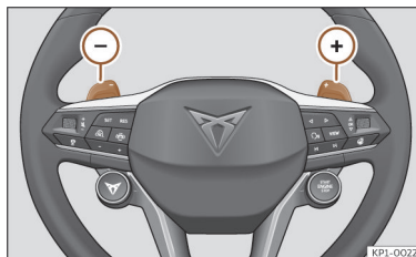
Afb. 120 Stuur: hendels voor automatisch schakelen.
