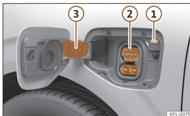
Afb. 61 Achter de laadklep van de accu, rechtsachter: laadcontactdoos.
