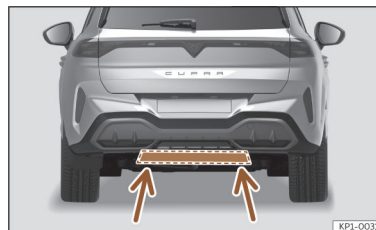
Afb. 86 Detectiegebied van de onderste sensor
