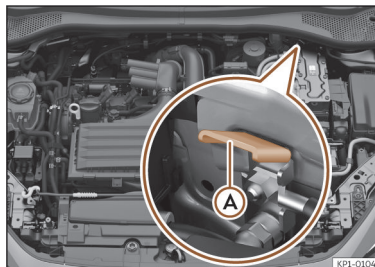
Afb. 209 In de motorruimte: aansluiting voor starthulp (massapunt).
