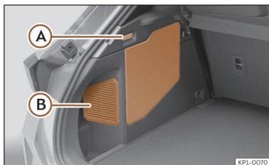
Afb. 233 Hybride wagens (PHEV): locatie van de accu in de bagageruimte
