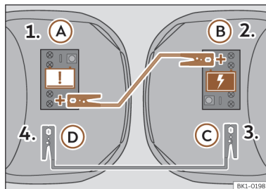
Afb. 210 Schakelschema van de startkabels.
