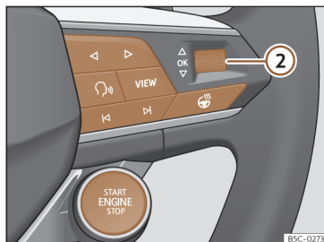
Afb. 92 Bedieningselementen aan het stuurwiel.
