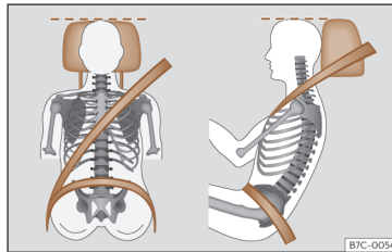
Afb. 25 Juist verloop van de gordelband en een juiste stand van de hoofdsteen van voren en opzij gezien.
