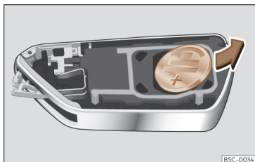
Afb. 73 Autosleutel: batterij verwijderen.
