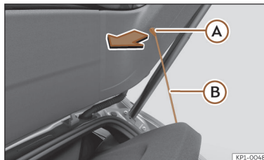
Afb. 182 In de bagageruimte: hoedenplank uit- en inbouwen.
