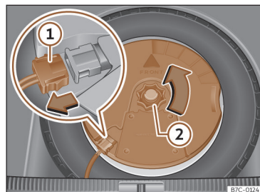
Afb. 240 In de bagageruimte: subwoofer uitbouwen.
