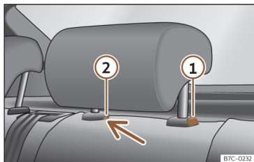
Afb. 98 Hoofdsteun achterin: verwijderen.
