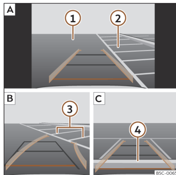
Afb. 161 Weergave op het scherm van het infotainmentsysteem: parkeren met de achteruitrijhulp.
