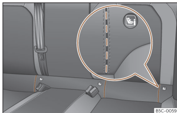
Afb. 37 Achterstoel: gestante gleuven voor toegang tot de ISOFIX/i-Size-bevestigingsbeugels.
