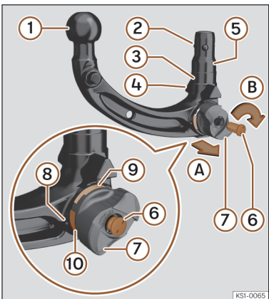
Afb. 175 Overzicht: verwijderbare trekhaak voor aanhangwagen.
