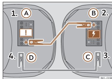
Afb. 182 Schakelschema van de startkabels.
