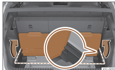
Afb. 165 In de bagageruimte: de tweede bodem van de bagageruimte vastzetten.
