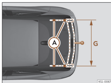
Afb. 173 Trekhaak: maten en bevestigingspunten.
