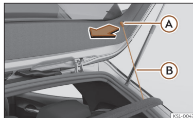
Afb. 161 In de bagageruimte: hoedenplank uit- en inbouwen.
