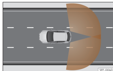
Afb. 112 Detectiegebieden van de sensoren.
