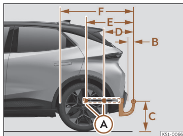
Afb. 172 Trekhaak: maten en bevestigingspunten.
