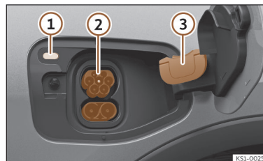
Afb. 57 Achter de laadklep van de accu, rechtsvoor: laadcontactdoos.
