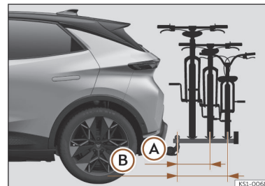
Afb. 171 Schematische voorstelling van de maximale overhang van de lading in een fietsendrager voor twee of drie fietsen.
