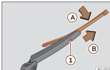
Afb. 180 Ruitenwisserblad van achterraut vervangen.
