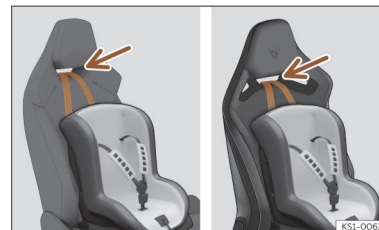
Afb. 43 Bijrijdersstoel: afstelling en montage volgens de Top Tether-gordel.
