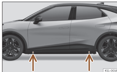
Afb. 205 Steunpunten voor de krik.
