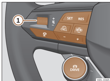
Afb. 80 Bedieningselementen aan het stuurwiel.
