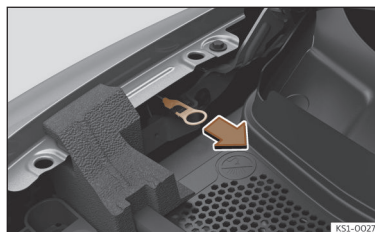
Afb. 60 Tussen het spatscherm rechts en het scharnier van de voorruimte: Hendel voor handmatige noodontgrendeling van de laadsteker.
