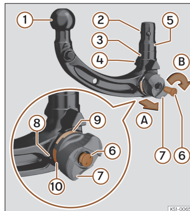
Afb. 174 Overzicht: verwijderbare trekhaak voor aanhangwagens.
