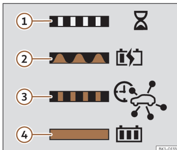
Afb. 60 Aan de binnenkant van de klep van de laadaansluiting: sticker met informatie over de indicator van het laadproces.
