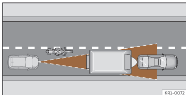
Afb. 139 Motorrijder die voor u rijdt, buiten de actieradius van de radarsensor.
