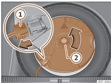
Afb. 240 In de bagageruimte: subwoofer uitbouwen.
