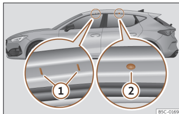
Afb. 201 Bevestigingspunten voor de reling van het dakdragersysteem (Leon).
