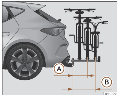
Afb. 205 Schematische voorstelling van de maximale overhang van de lading in een fietsendrager voor twee of drie fietsen.
