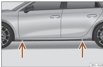
Afb. 244 Steunpunten voor de krik.
