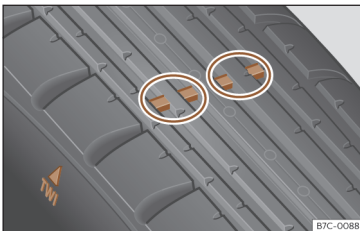
Afb. 237 Bandenprofiel: slijtagemerkttekens.
