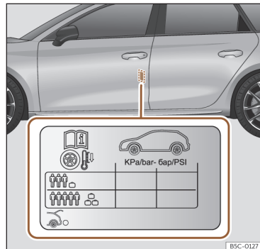
Afb. 236 Plaats van de sticker van de bandenspanningen.
