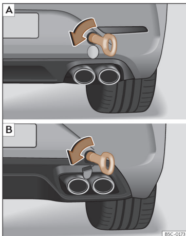
Afb. 218 Aan de rechterzijde van de achterbumper: vastgeschroefd sleepoog. A Leon Sportstourer; B Leon.
