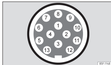
Afb. 202 Schematische weergave: toewijzing van de pinnen van het stopcontact voor de aanhangwagen.
