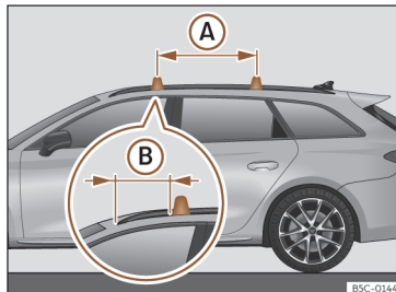
Afb. 200 Bevestigingspunten voor de reling van het dakdragersysteem (Leon Sportstourer).
