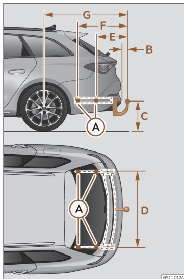
Afb. 206 Maten en bevestigingspunten voor het achteraf inbouwen van een trekhaak.
