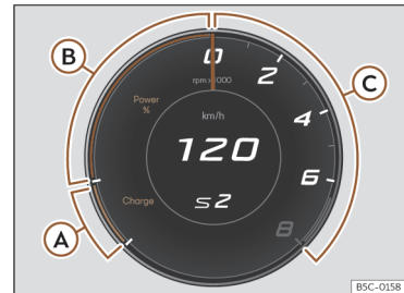
Afb. 7 Digitaal instrumentenpaneel: Powermeter (Cupra-weergave)
