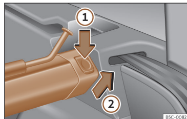
Afb. 190 In de bagageruimte: scheidingsnet uitbouwen.
